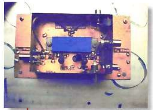
Eindtrap met coaxiale schakelaars voor 60 cm
